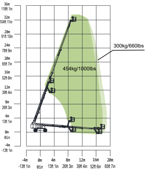
Zakres ruchu i zasięgów ZT32J-V
